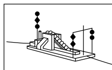
Manövriertes Fahrzeug bei Bagger- oder Unterwasserarbeiten; Passierseite: 2 grüne Lichter bzw. 2 schwarze Rhomben
